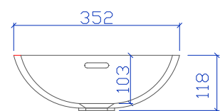
Schnitt-vorne
