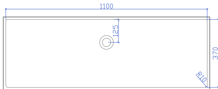
Ansicht-oben
