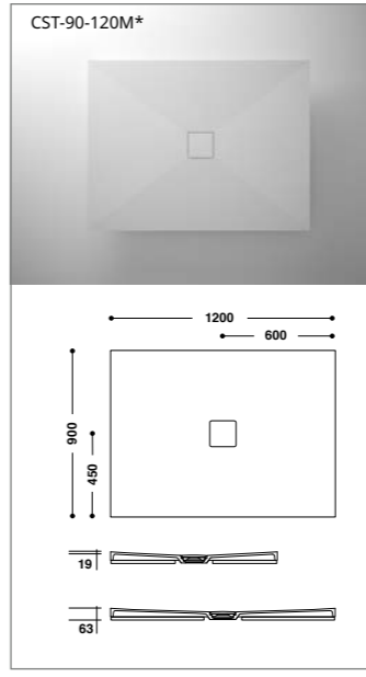
* Mittleres Abflussloch
