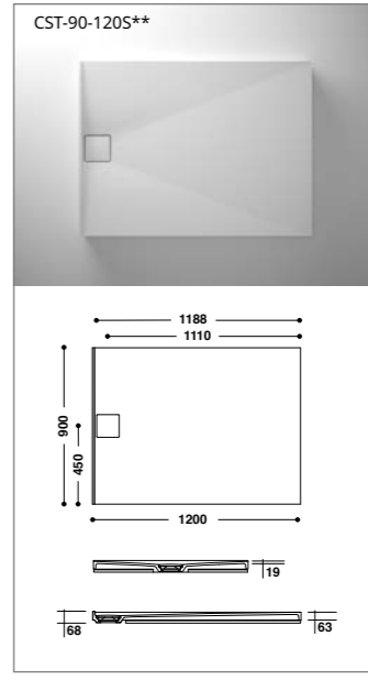
** Seitliches Abflussloch
